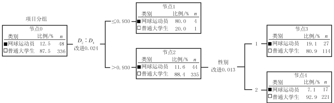
图2 分类树结构
