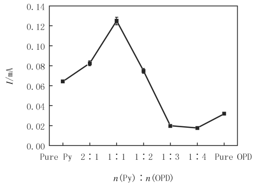
图5 峰电流随n(Py) : n(OPD)的变化
