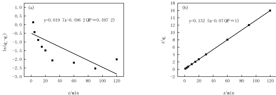
图6 准一级动力学拟合曲线(a)和准二级动力学拟合曲线(b)
