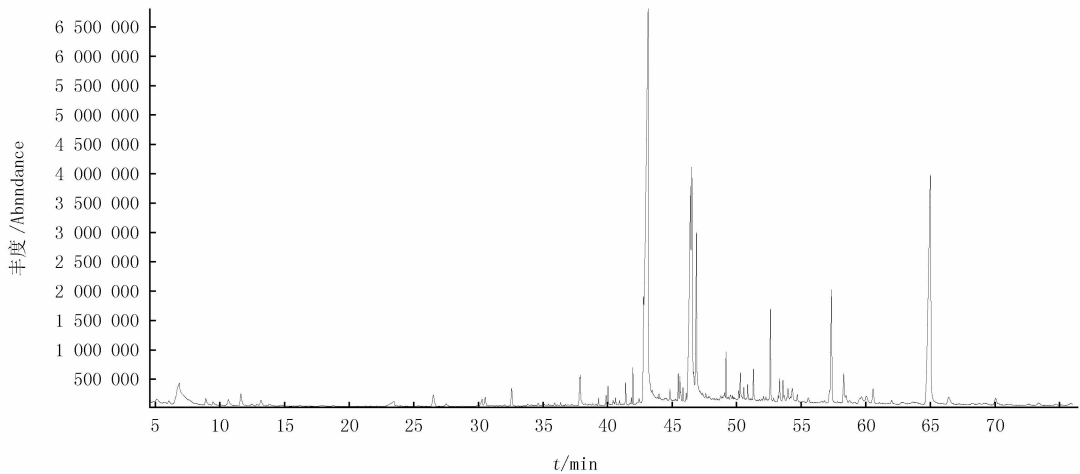
图5 金银花挥发油总离子流色谱图
