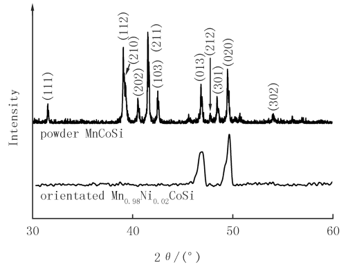
图2 强磁场凝固后的 \text{Mn}_{0.98}\text{Ni}_{0.02}\text{CoSi} 合金样品的室温 XRD 图谱
