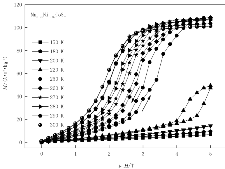
图3 强磁场凝固后的 \text{Mn}_{0.98}\text{Ni}_{0.02}\text{CoSi} 合金样品的等温磁化曲线
