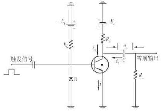
图3 三极管雪崩电路
