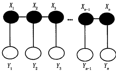
图 1 线性结构的CRF模型
