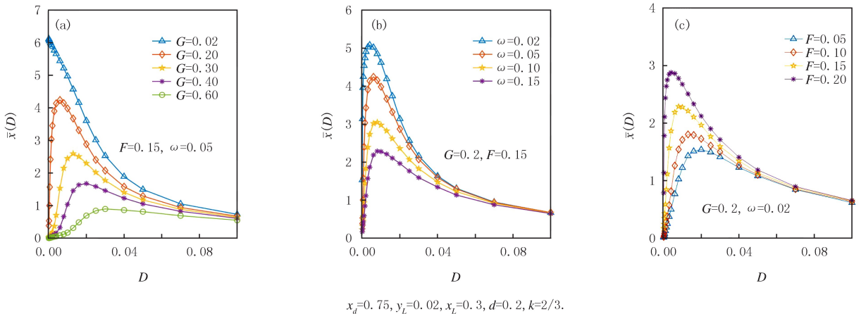
图4 不同参数对固定T形结构中熵随机共振的影响
