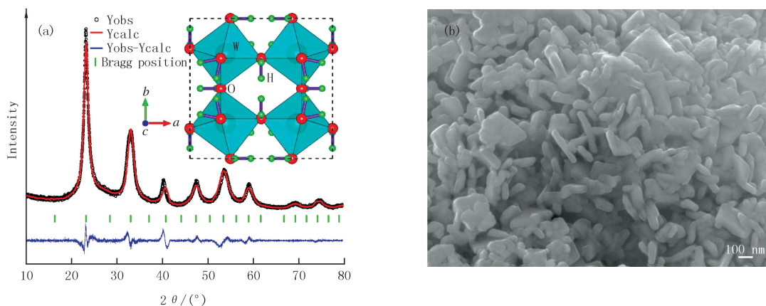
图3 氢钨青铜 H_{0.25}WO_3 的 Rietveld 精修图谱和沿 c 轴投影的晶体结构示意图 (a) 以及 SEM 照片 (b)
