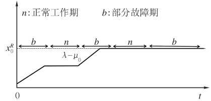
图2 \lambda = \mu_1 时 X(t) 随时间 t 的变化
