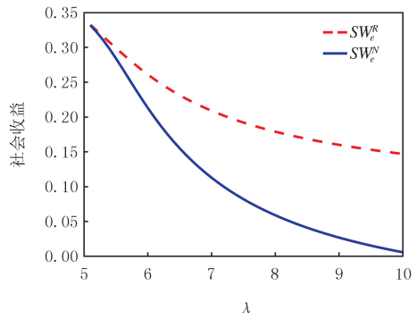
图6 均衡社会收益随到达率 lambda 的变化曲线 Fig. 6 SW_e^R and SW_e^N versus \lambda
