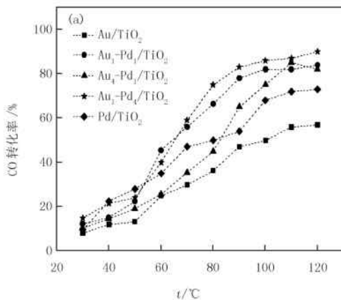
图4 不同钯金比例催化剂在 CO 氧化反应的活性图 (a) 及催化剂 Au 1 -Pd 4 /TiO 2 的循环实验图 (b)
