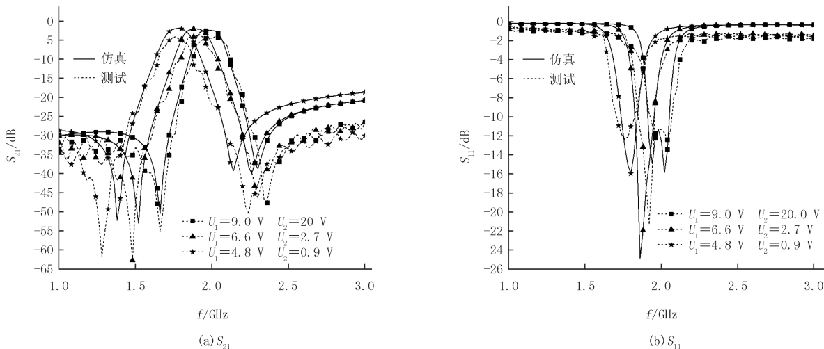
图 10 滤波器低频带的仿真和测试结果
