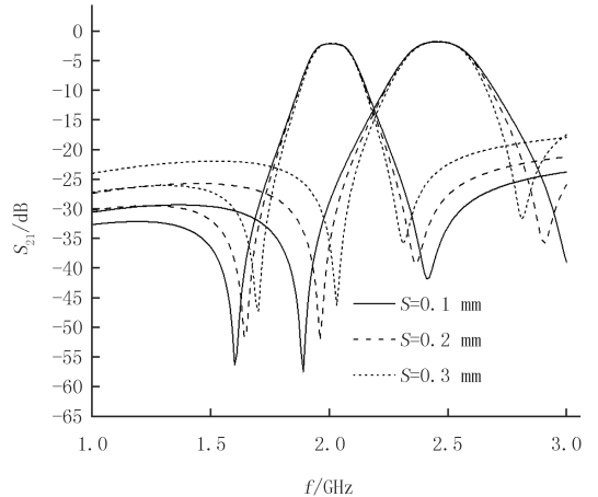
图 8 S 对滤波器传输零点的影响
