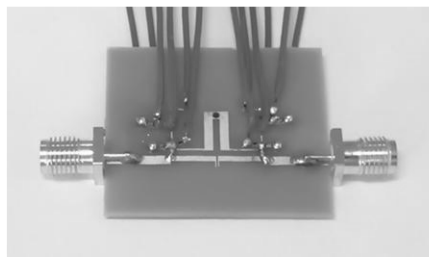
图 9 滤波器实物图
