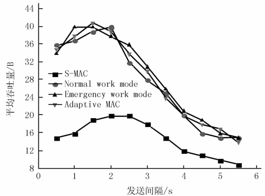
图17 面状拓扑,网络吞吐量比较
