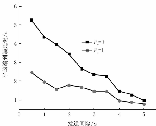
图9 普通工作模式端到端延时
