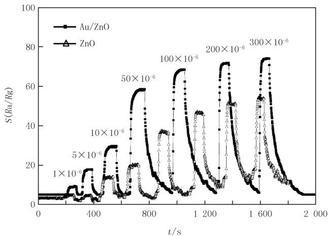
图 6 ZnO、Au/ZnO 纳米材料在不同丙酮体积分数下的响应曲线
