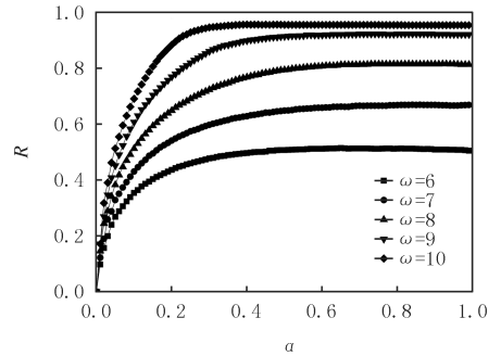
图6 全连通网络中,不同 \omega 下, R 随 \alpha 的变化关系
