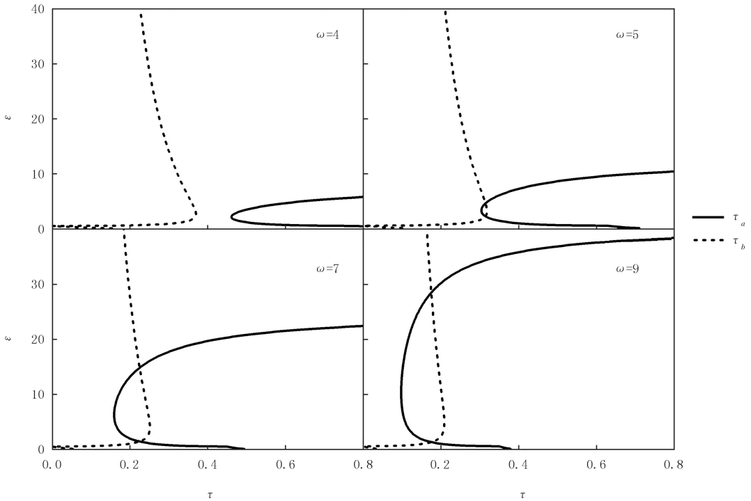
图1 不同 \omega 下, 耦合振子系统在参数空间中 \epsilon - \tau 的振幅死亡区域
